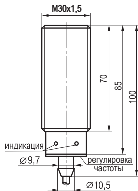
Габаритный чертёж
