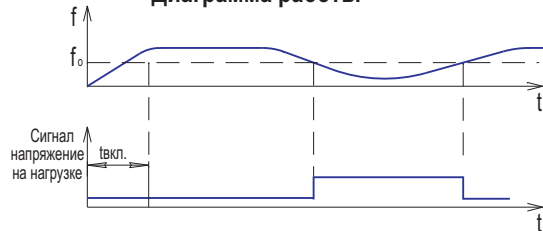
Диаграмма работы
